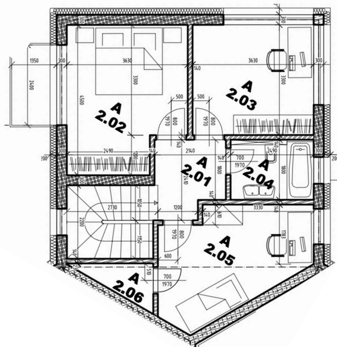
Podlažie č. 2
